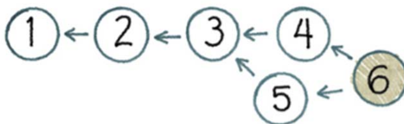
Фигура 5: Разпределена система за следене на версиите - Модел за следене на историята
